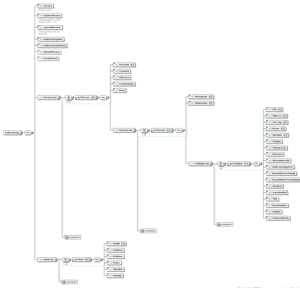
Figur 2. XML Schema.
